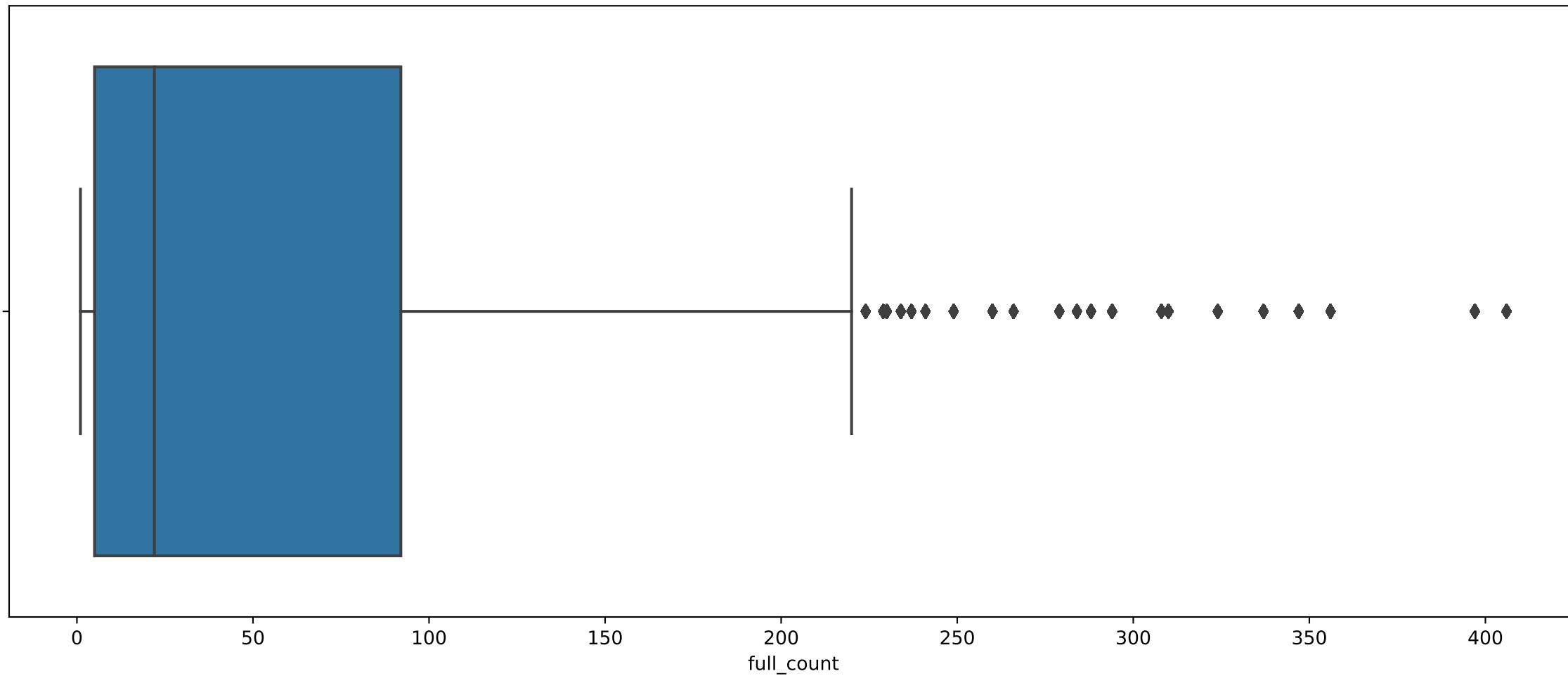
hyper : Boîte à moustache (fréquences absolues, 90% quantile)
