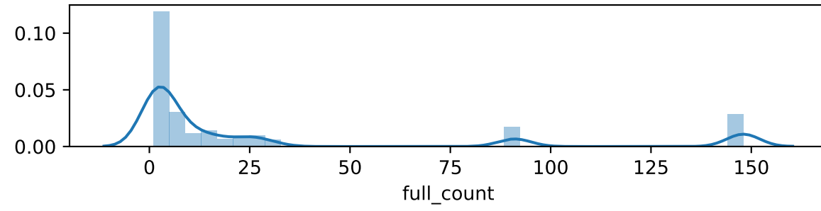
archi : 90% quantiles
