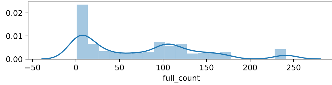
maxi : 90% quantiles
