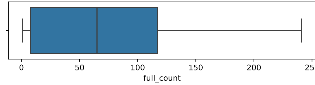
maxi : 90% quantiles
