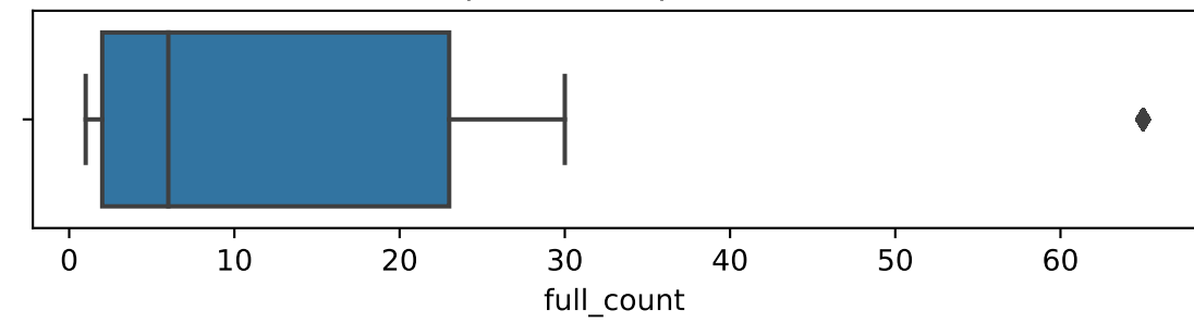
hypra : 90% quantiles
