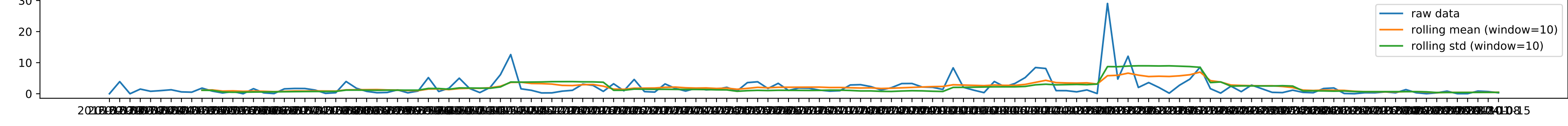
supra
