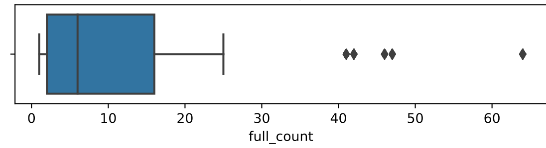
supra : 90% quantiles
