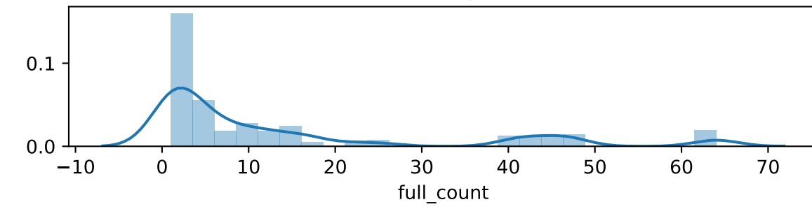
supra : 90% quantiles
