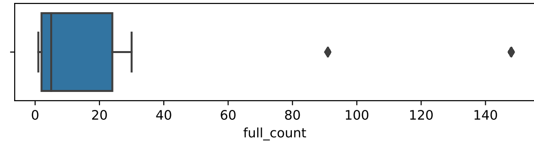
archi : 90% quantiles
