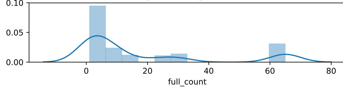
hypra : 90% quantiles
