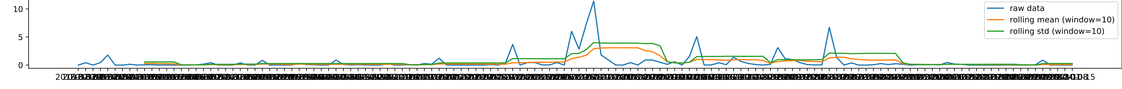
hypra
